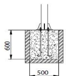
Cimentación
